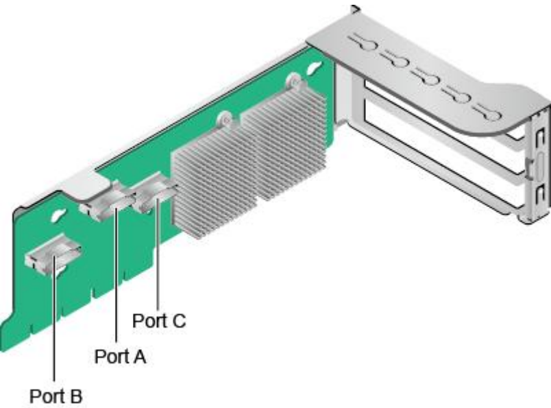
图 5-24 12NVMe 专用 Riser 卡 3
