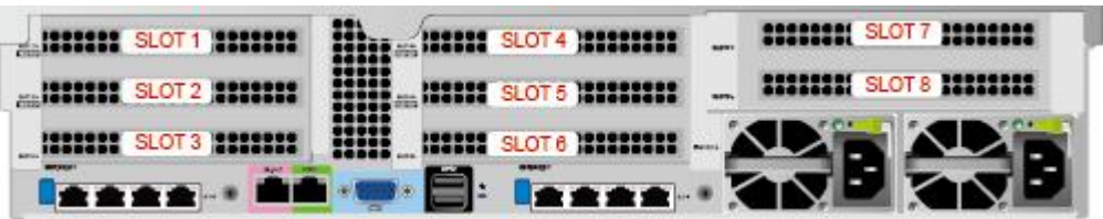
图 5-30 PCIe 插槽
