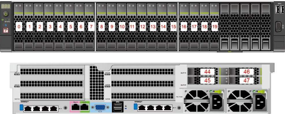
图 5-17 8x2.5 SAS/SATA+12x2.5 NVMe 硬盘配置硬盘编号
