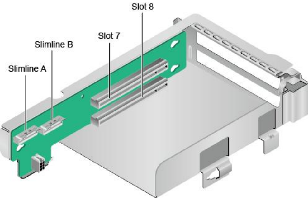
图 5-28 2x8 Riser 卡 7
