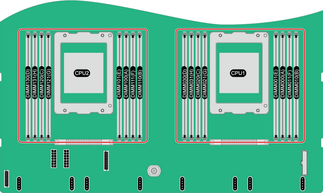
图 5-21 内存槽位编号
