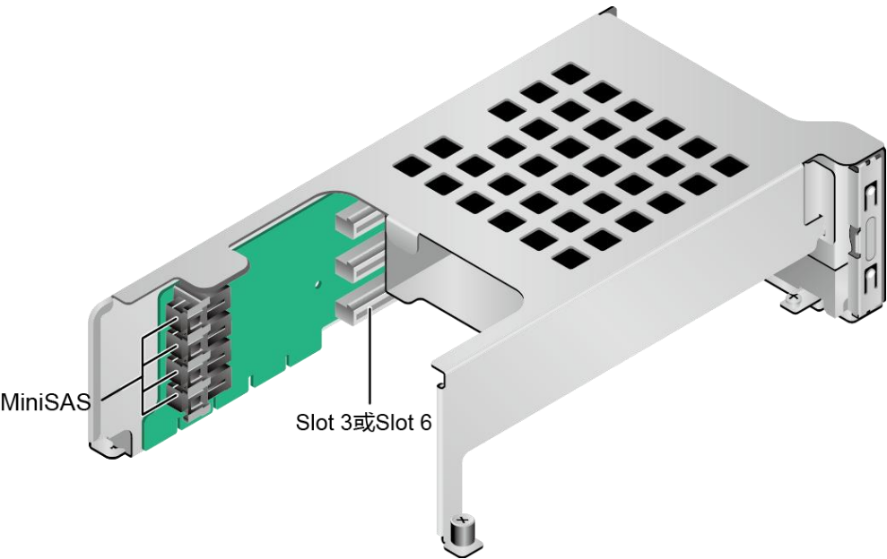
图 5-27 SAS Riser 卡 6
