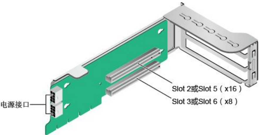
图 5-23 1x8+1x16 Riser 卡 2
