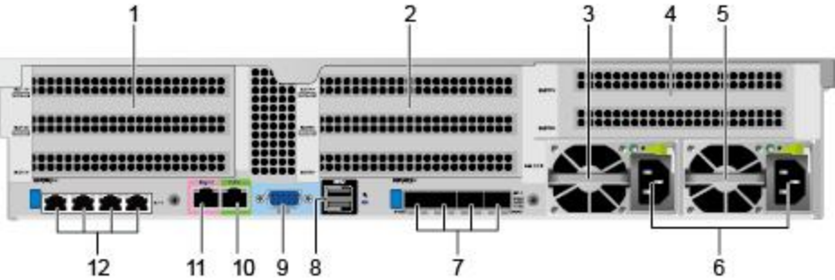
图 5-9 后面板组件
