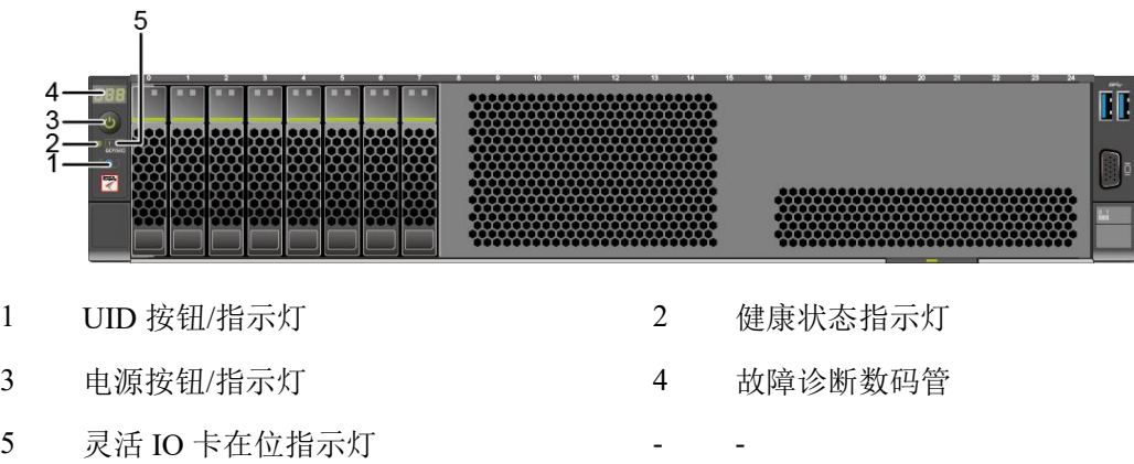
图 5-8 8x2.5 英寸硬盘配置前面板指示灯和按钮
