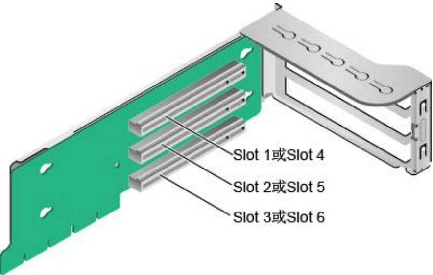
图 5-22 3x8 Riser 卡 1
