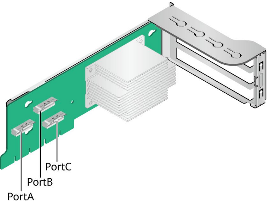
图 5-25 12NVMe 专用 Riser 卡 4
