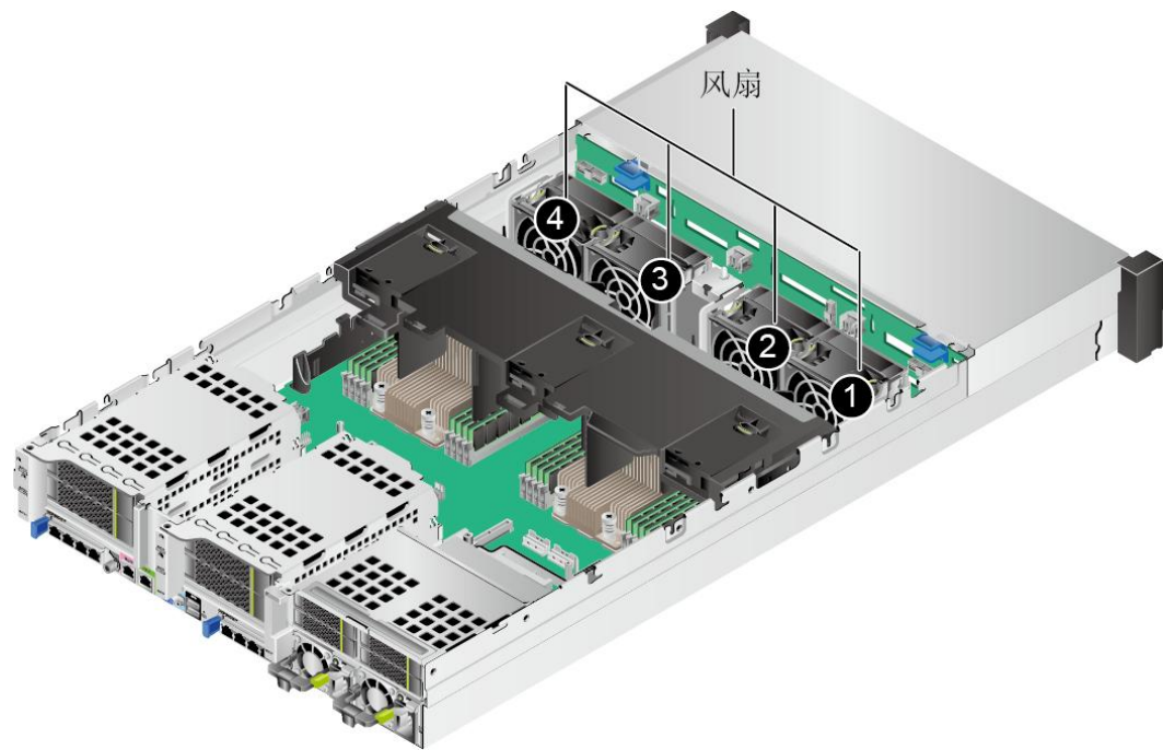
图 5-31 风扇位置图
