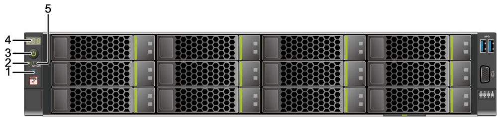
图 5-5 12x3.5 英寸硬盘配置前面板指示灯和按钮
