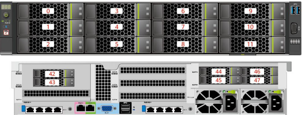
图 5-15 12x3.5 英寸硬盘 RAID 直通配置
