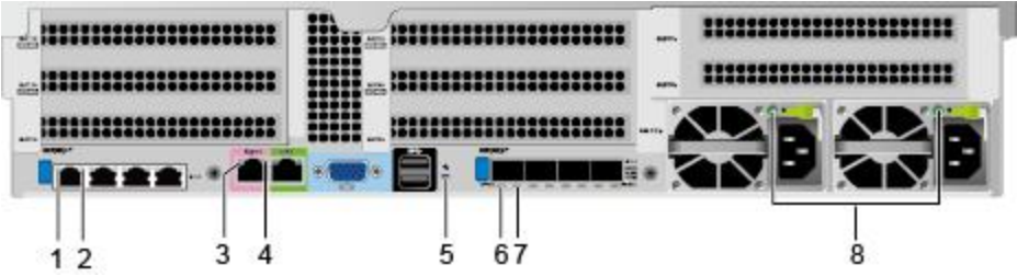
图 5-10 后面板指示灯
