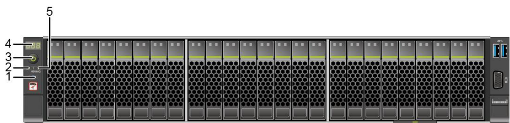
图 5-6 25x2.5 英寸硬盘配置前面板指示灯和按钮
