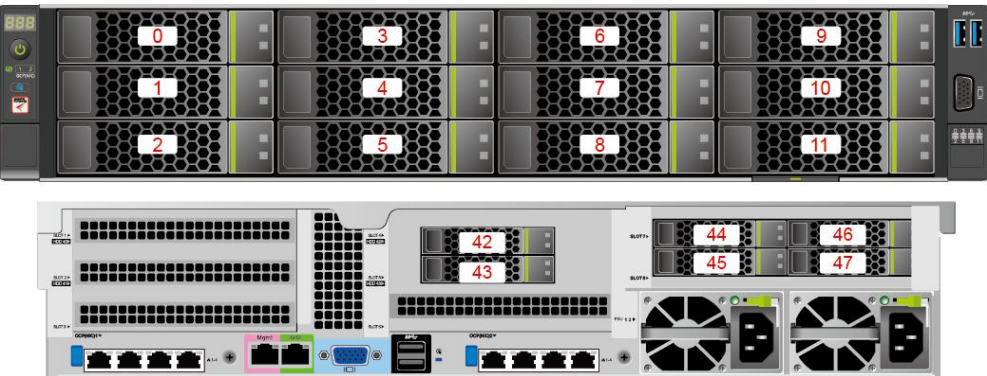
图 5-14 12x3.5 英寸硬盘直通配置
