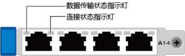
图 5-11 TM210（4xGE 电口）
