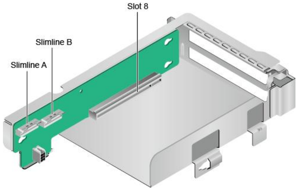
图 5-29 1x16 Riser 卡 8
