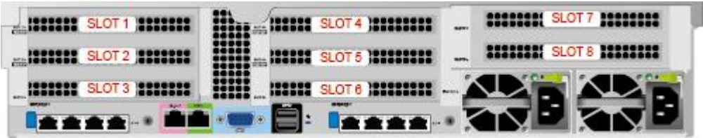
图 5-35 PCIe 插槽
