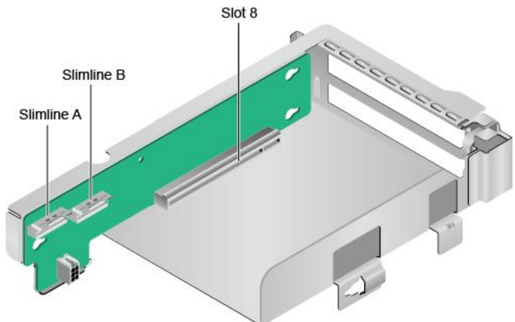
图 5-34 1x16 Riser 卡 7
