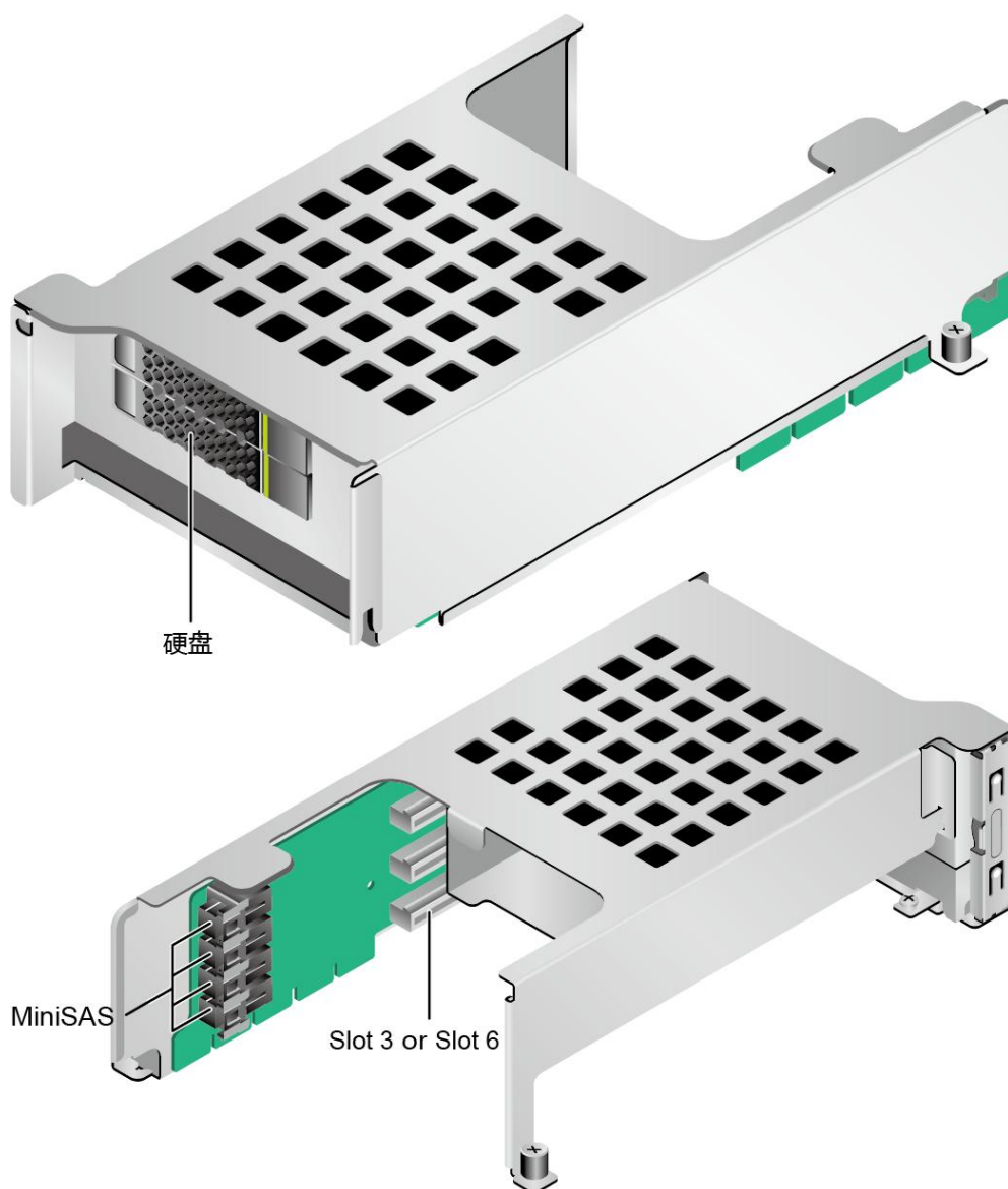
图 5-32 SAS Riser 卡 5
