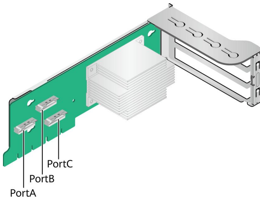
图 5-30 12NVMe 专用 Riser 卡 3
