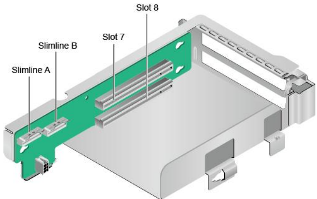
图 5-33 2x8 Riser 卡 6
