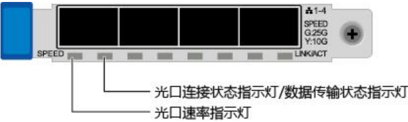
图 5-16 TM280（4x25GE 光口）
