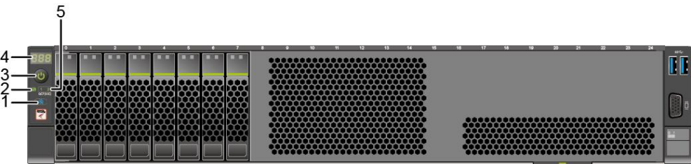
图 4-13 8x2.5 英寸硬盘配置前面板指示灯和按钮
