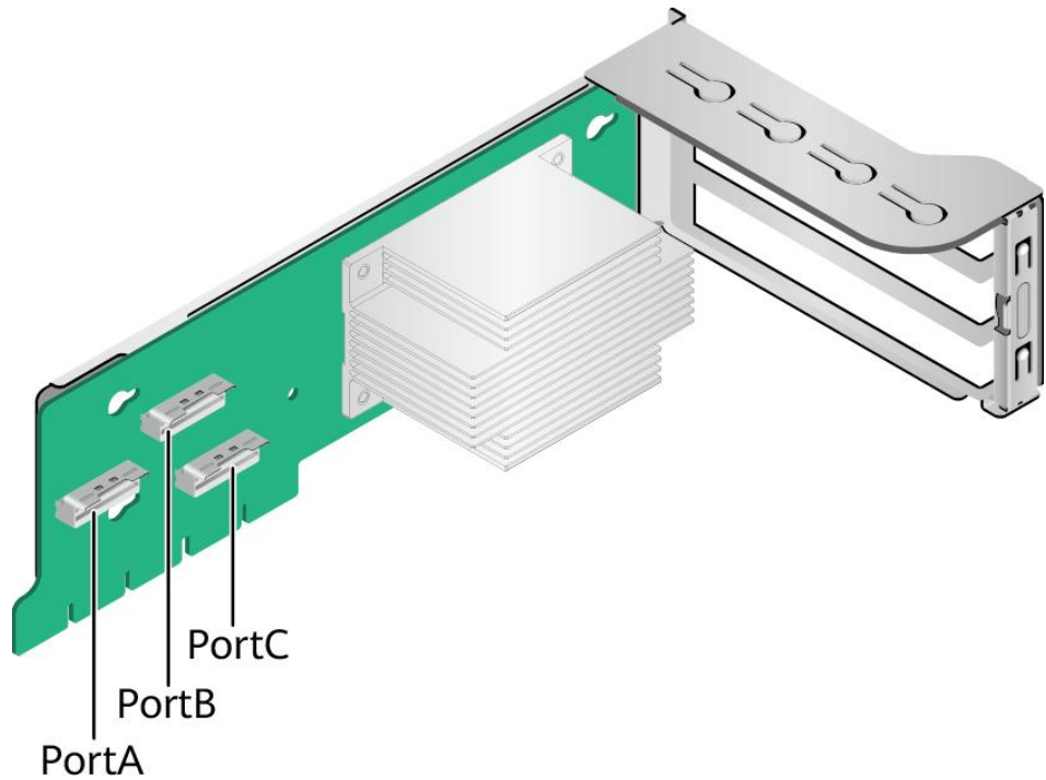
图 4-23 Riser 卡 4
