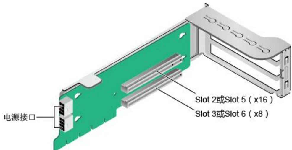
图 4-20 Riser 卡 2（1x8+1x16）
