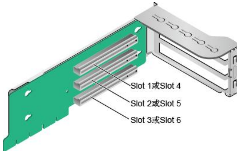
图 4-19 Riser 卡 1（3x8）
